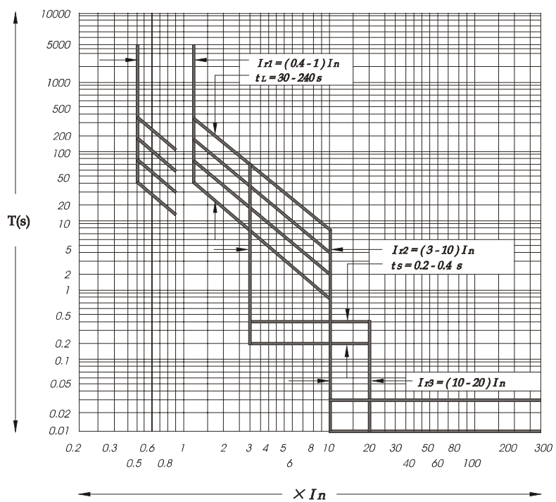
Время-токовая характеристика для ВА-730, расцепитель типа L
