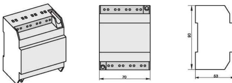
10.2.4. Блок питания БП-730/750 и модуль передачи сигналов МПС-730/750
