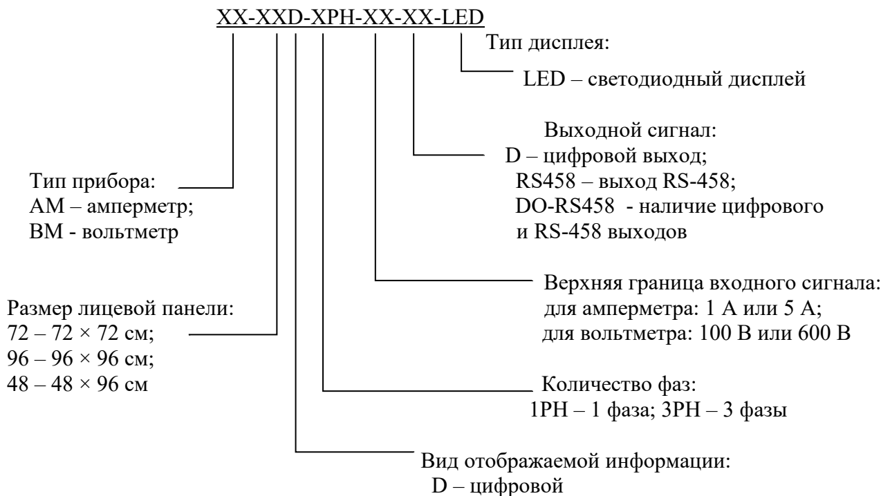
Рисунок 1 – Структурная схема обозначения модификаций амперметров и вольтметров
